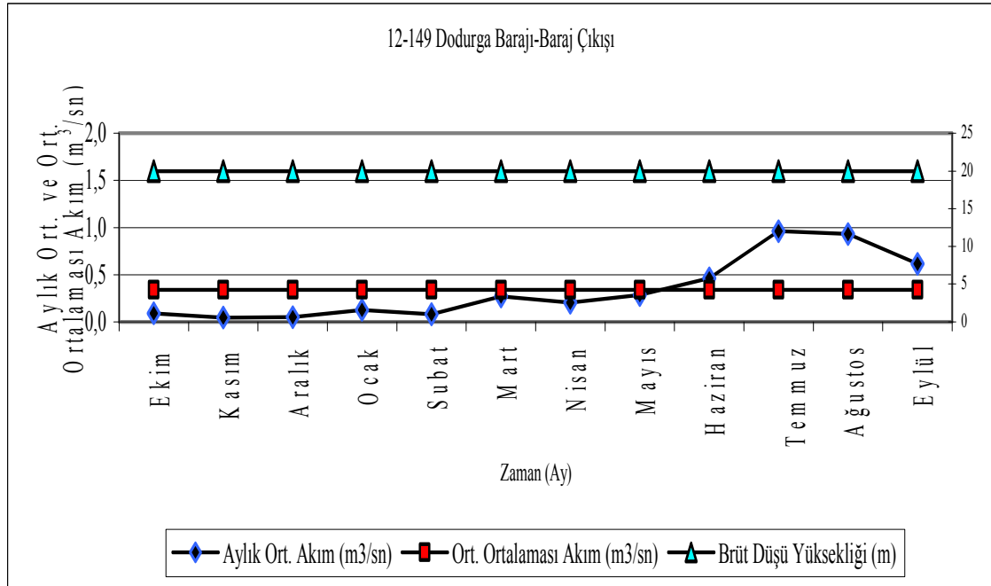
Şekil 3 (Devamı). Porsuk Havzasındaki barajlara ait ortalama aylık akım değerleri (m³/sn).
