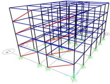
Şekil 5: Kısmi duvarlı analitik model.
