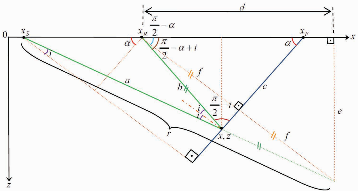
Fay düzleminde gelen yansıma için sismik ışın geometrisi.
