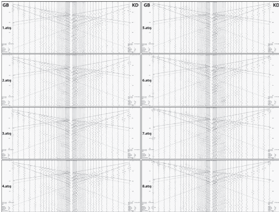
Şekil 12. Atışlara ait sismik profil ayrıntısı (Soldaki ortak-uzaklık sismik yansıma kesiti fayın güneybatı bloğundan, sağdaki ortak-uzaklık sismik yansıma kesiti fayın kuzeydoğu bloğundan elde edilmiştir).
