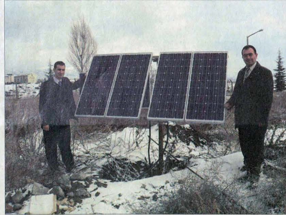
Yard. Doç. Dr. Mehmet Kurban (sağda) ve Araş. Gör. Fatih Onur Hocaoğlu tarafından kurulan sistem 10 metrelik bir rüzgar türbininden ve 8 adet güneş panelinden oluşuyor. İki sistem birlikte çalıştırılarak üretilen enerjinin sürekliliği sağlanıyor.
