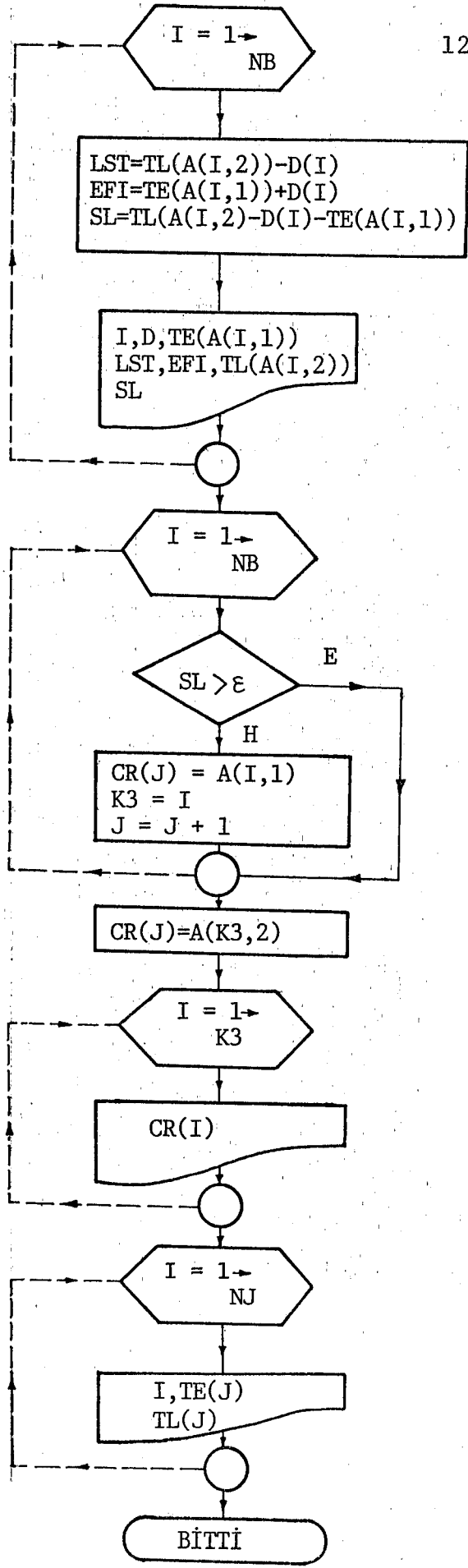
ŞEKİL 43 : KEPİR Programı Akış Diagramı.
