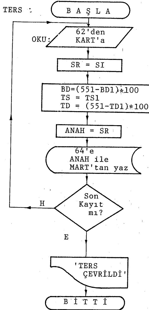
ŞEKİL 27 : TERS Programının Akış Diyagramı.
