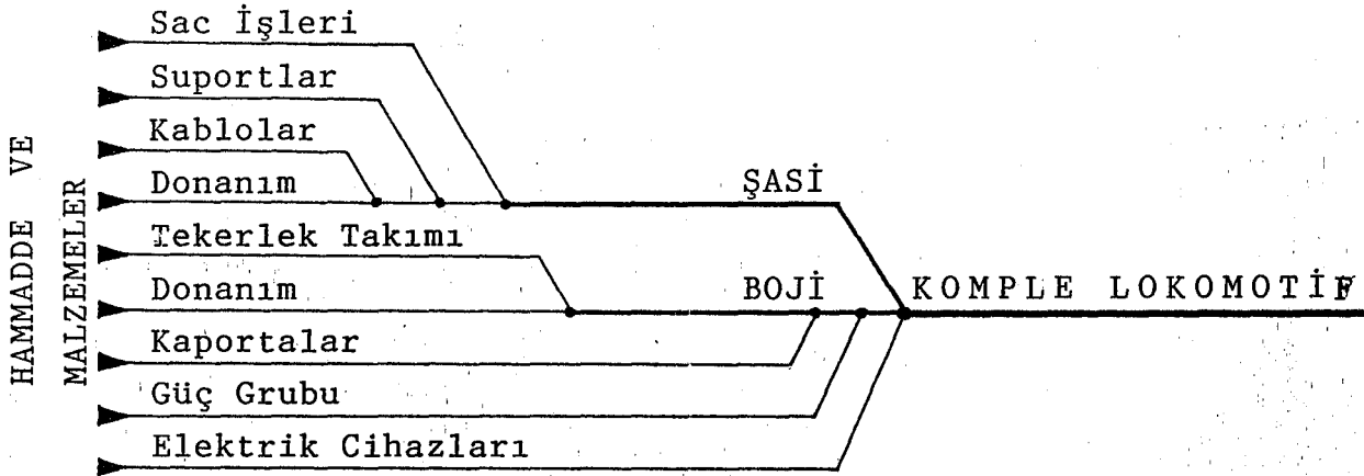
ŞEKİL 7 : Birleştirme Süreçli Üretime Bir Örnek
