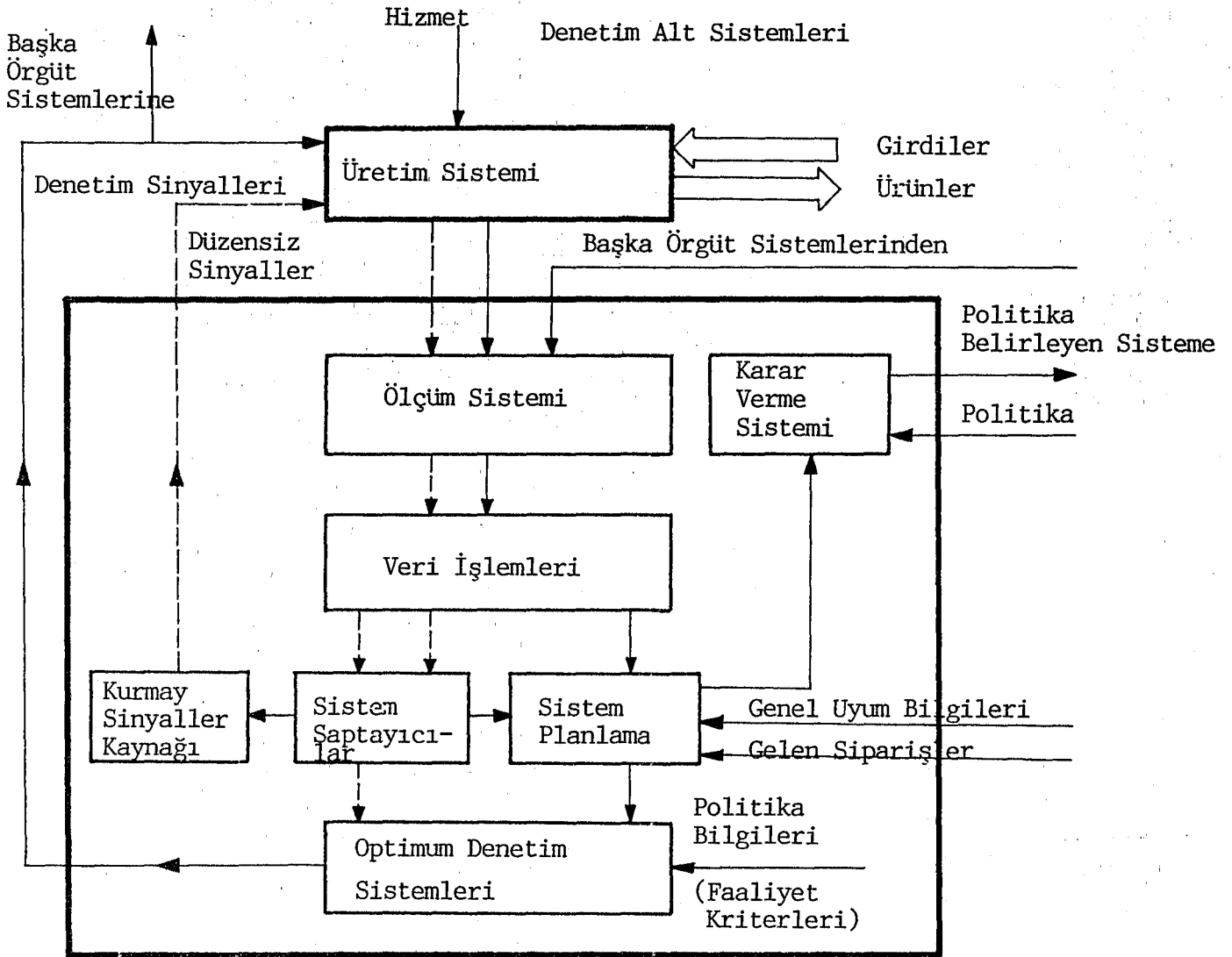
ŞEKİL 3 : Denetim Altsistemleri ile İlişkili Üretim Sistemi.
