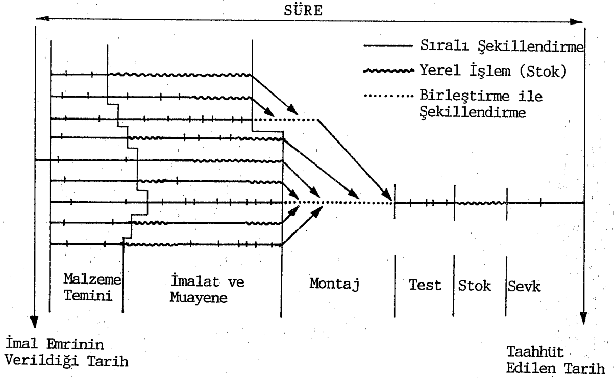
ŞEKİL 19 : Bir Mamül İçin İmalat Faaliyetlerinin Şematik Gösterimi. İşlemleri En Uzun Süren Parçaya Ait Sürelerin Toplanması İle İmalata Başlama Emrinden Taahhüt Edilmiş Gönderme Tarihin Kadar Olan Süre Hesaplanmış Olur.
