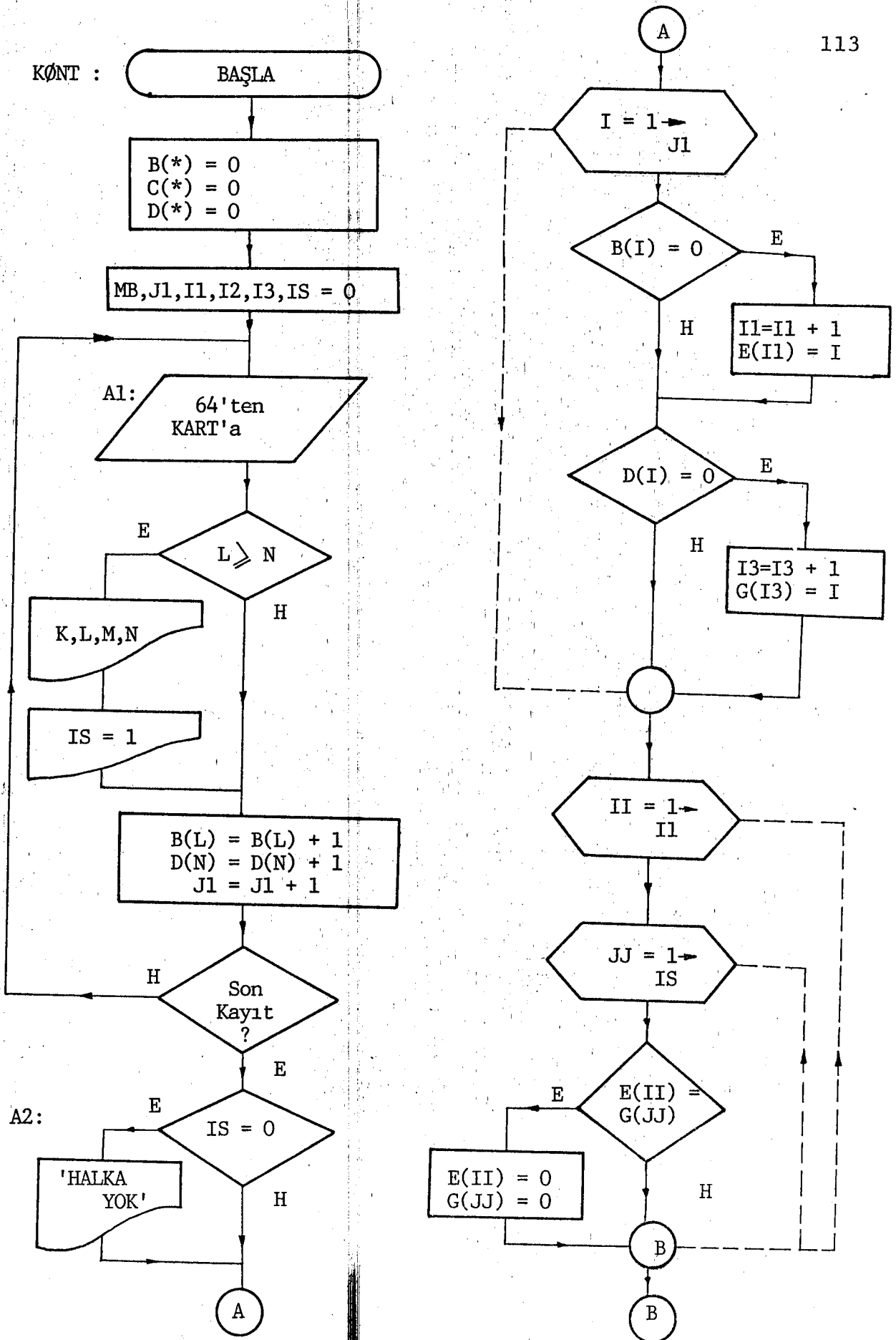
ŞEKİL 39 : KONT Programı Akış Diagramı
