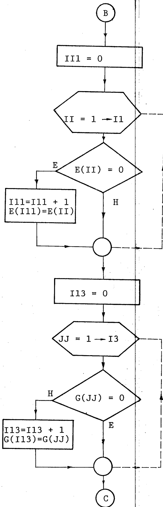
KONT Programı Akış Diagramı (Devam)
