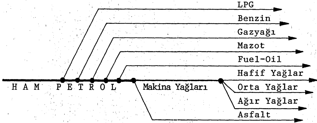
ŞEKİL 5 : Ayırma Yolu ile Yapılan Üretime Bir Örnek
