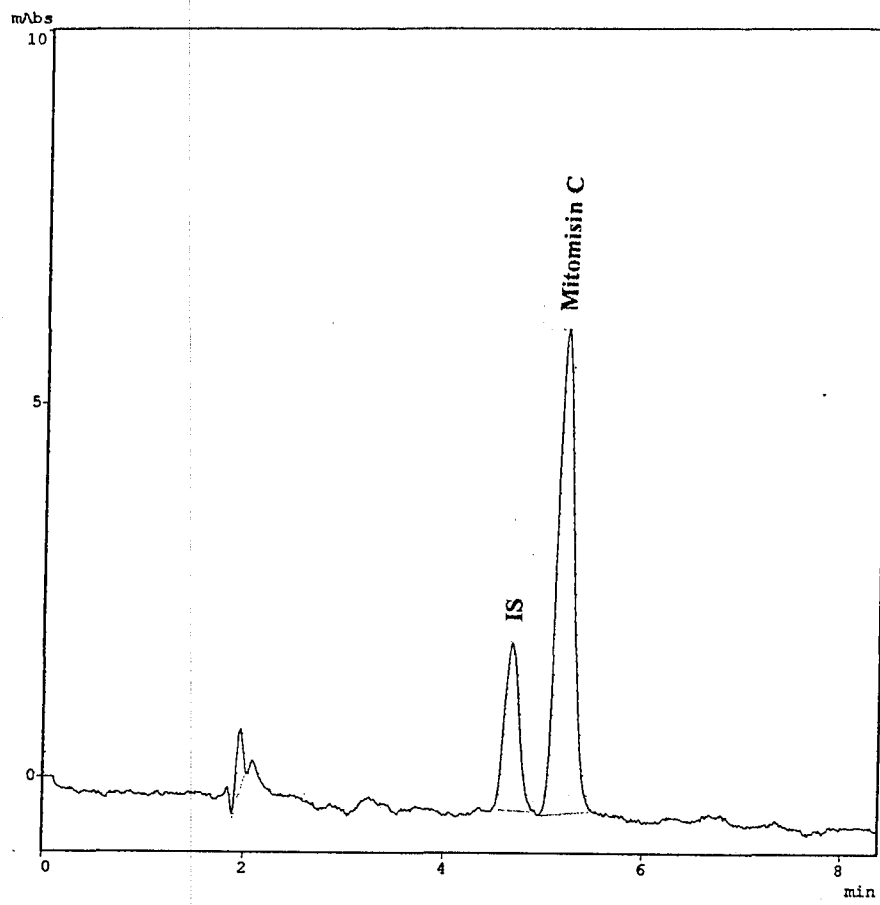
Şekil 4.3.1. Standart Mitomisin C ( 5.86 \times 10^{-6} \text{M} ) çözeltisinin IS varlığında kromatogramı
