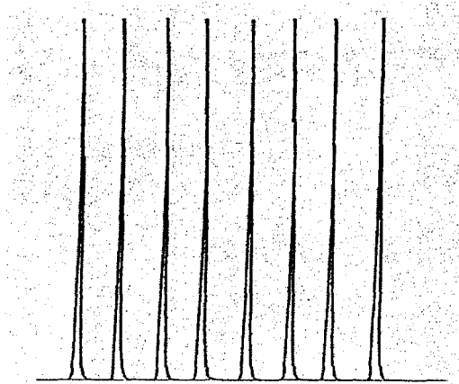
Şekil 4.1.2.1. Standart mitomisin C ( 1.0 \times 10^{-5} M) çözeltisinin 1.0 mL/dk akış hızında ve 363 nm' deki sinyallerinin tekraredilebilirliği.
