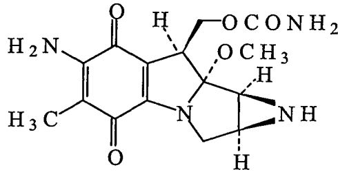
Şekil.2.1.1. Mitomisin C' nin kimyasal yapısı
