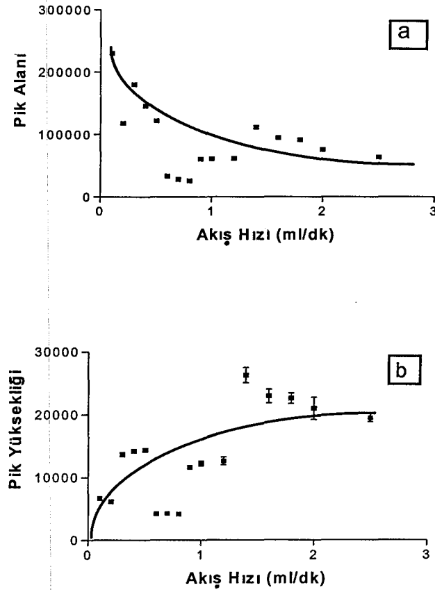
řekil 4.1.1.2. Akıř hızının mitomisin C sinyallerine etkisi pik alanı (a) ve pik yksekliđi (b).
